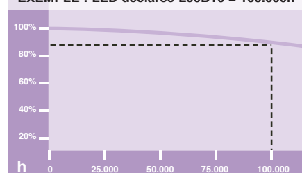
EXEMPLE : LED déclarée L90B10 = 100.000h
